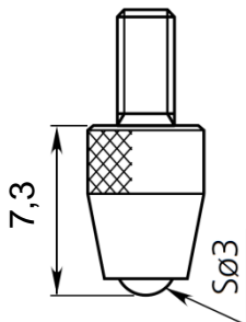
Standardní dotykové tělísko Obj.č. 901312
